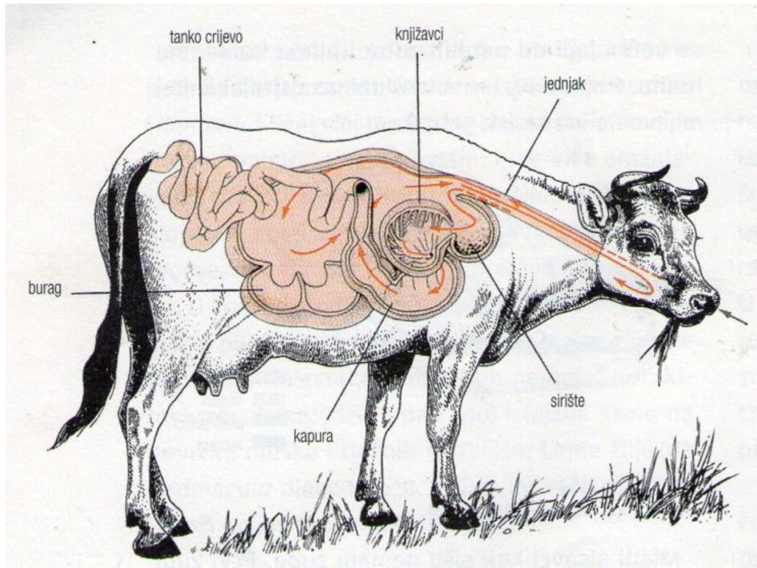
Želudac preživača
