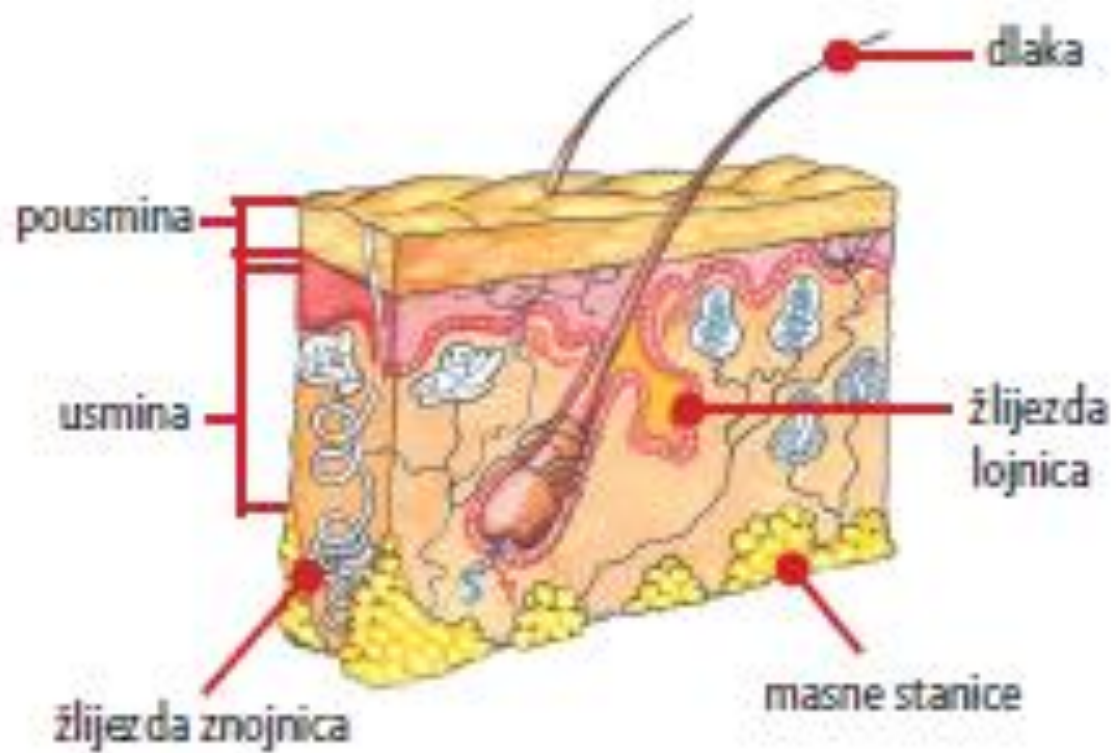
Koža sisavaca
